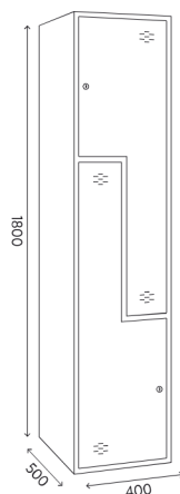
ARL-40-2P
