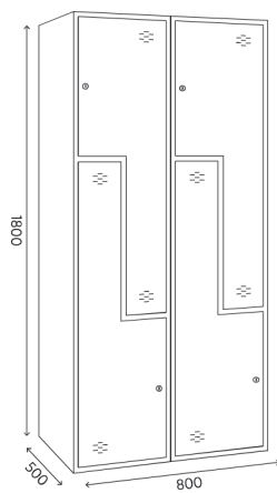
ARL-40-2P-2
