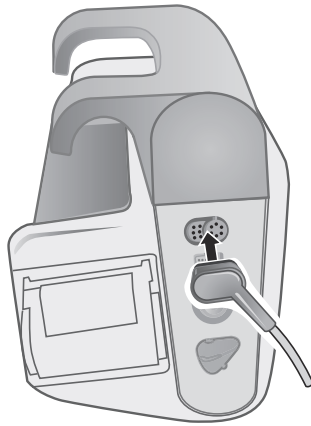
Figura 14-2 Conexión del cable de ECG de 12 derivaciones
