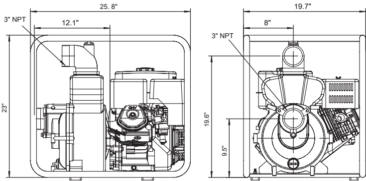
Figura 2 - Dimensiones para Modelos BA4C30AS
